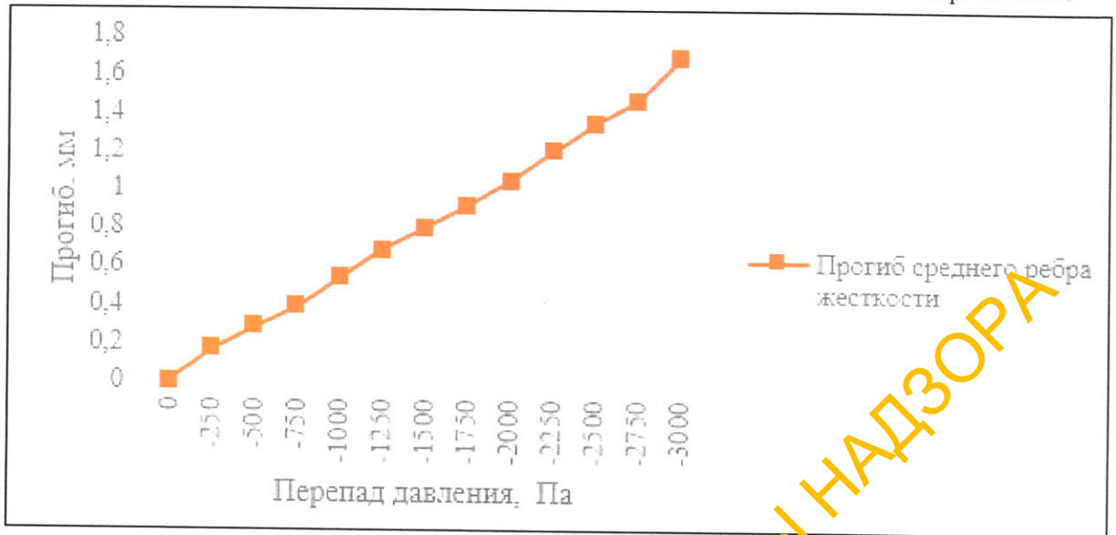
Рисунок 8 – График зависимости прогибов центрального пролета среднего ребра при воздействии отрицательных перепадов давления
